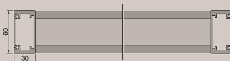
Horizontalschnitt: Maßstab 1:3
