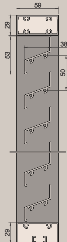
Vertikalschnitt: Maßstab 1:3
