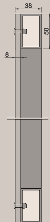
Vertikalschnitt: Maßstab 1:2
