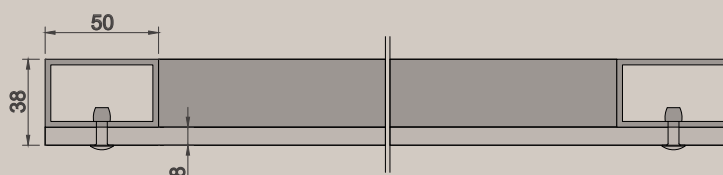
Horizontalschnitt: Maßstab 1:2
