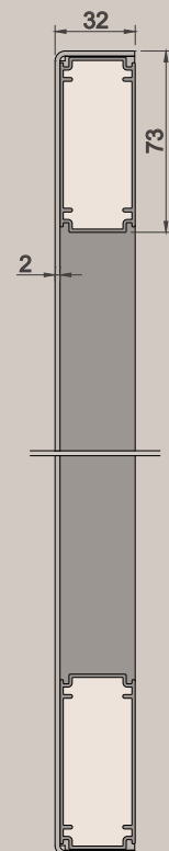
Vertikalschnitt: Maßstab 1:3
