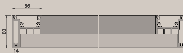
Horizontalschnitt: Maßstab 1:3
