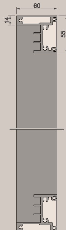
Vertikalschnitt: Maßstab 1:3
