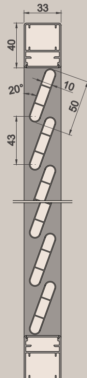
Vertikalschnitt: Maßstab 1:3
