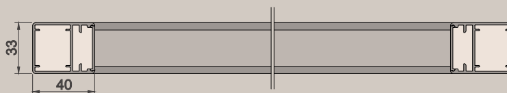
Horizontalschnitt: Maßstab 1:3
