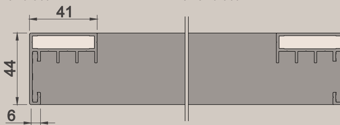
Horizontalschnitt: Maßstab 1:2
