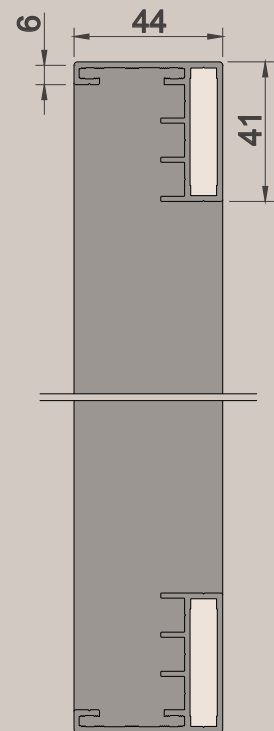
Vertikalschnitt: Maßstab 1:2
